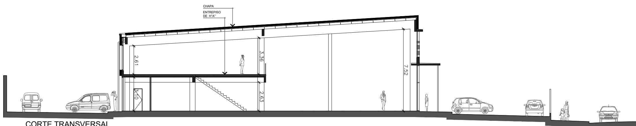
VISTA LATERAL
